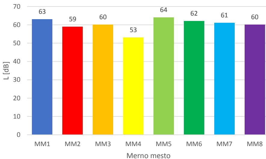
Slika 4.3. Ukupni nivo buke L_{den} – Mart 2020. godine
