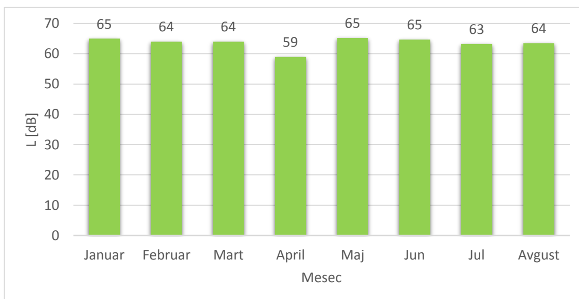
Slika MM5.6. Uporedni prikaz L_{den}
