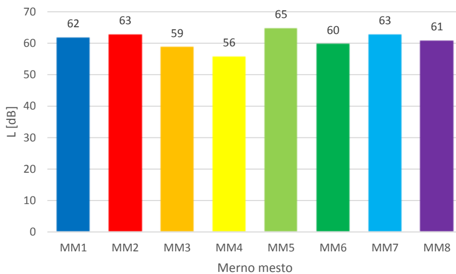
Slika 4.1. Ukupni nivo buke L_{den} – Januar 2020. godine
