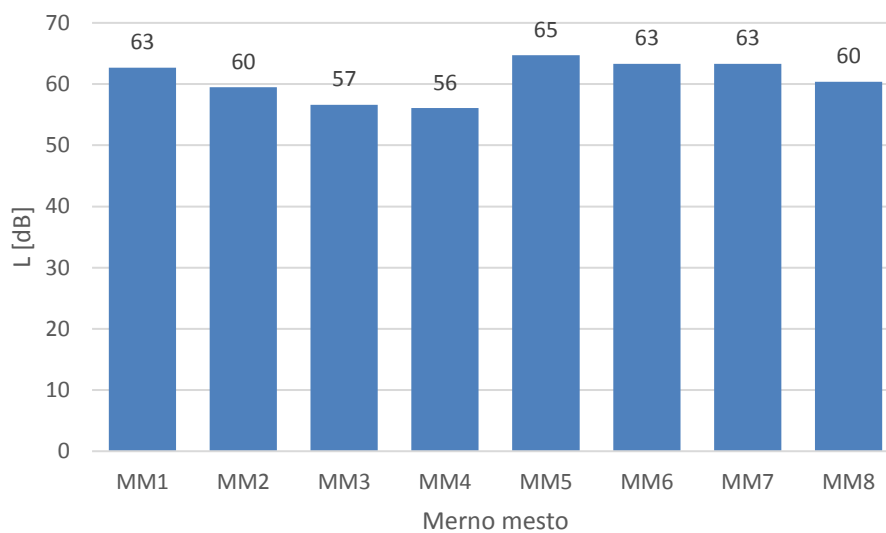
Slika 4.6. Ukupni nivo buke L_{den} – Jun 2020. godine
