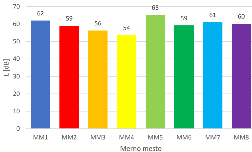
Slika 4.5. Ukupni nivo buke L_{den} – Maj 2020. godine
