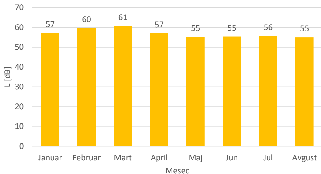
Slika MM3.3. Uporedni prikaz L_{day}
