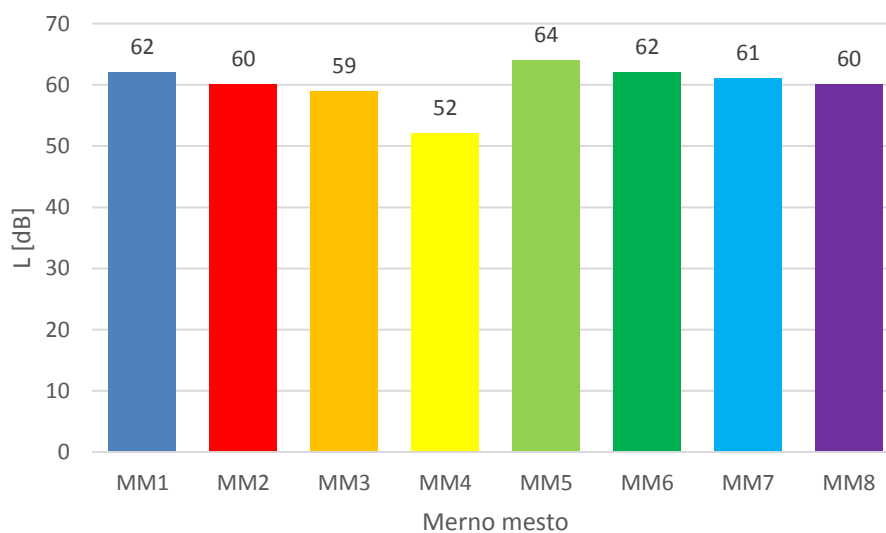
Slika 4.2. Ukupni nivo buke L_{den} – Februar 2020. godine
