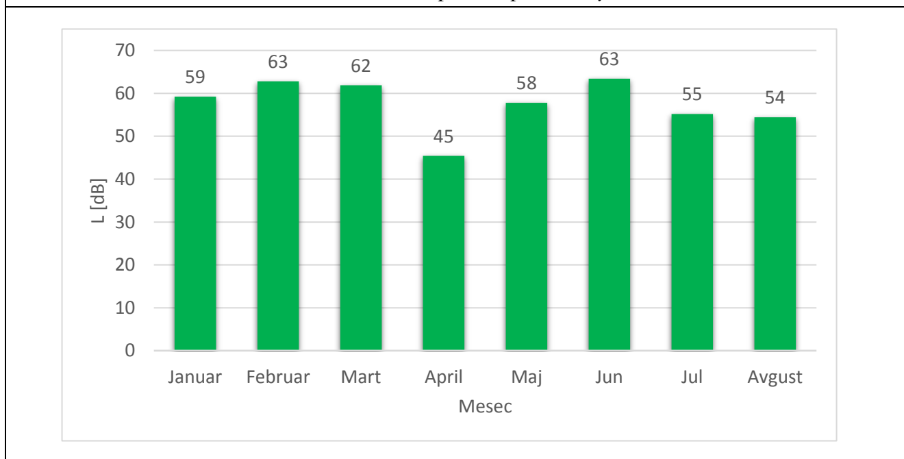
Slika MM6.4. Uporedni prikaz L_{evening}
