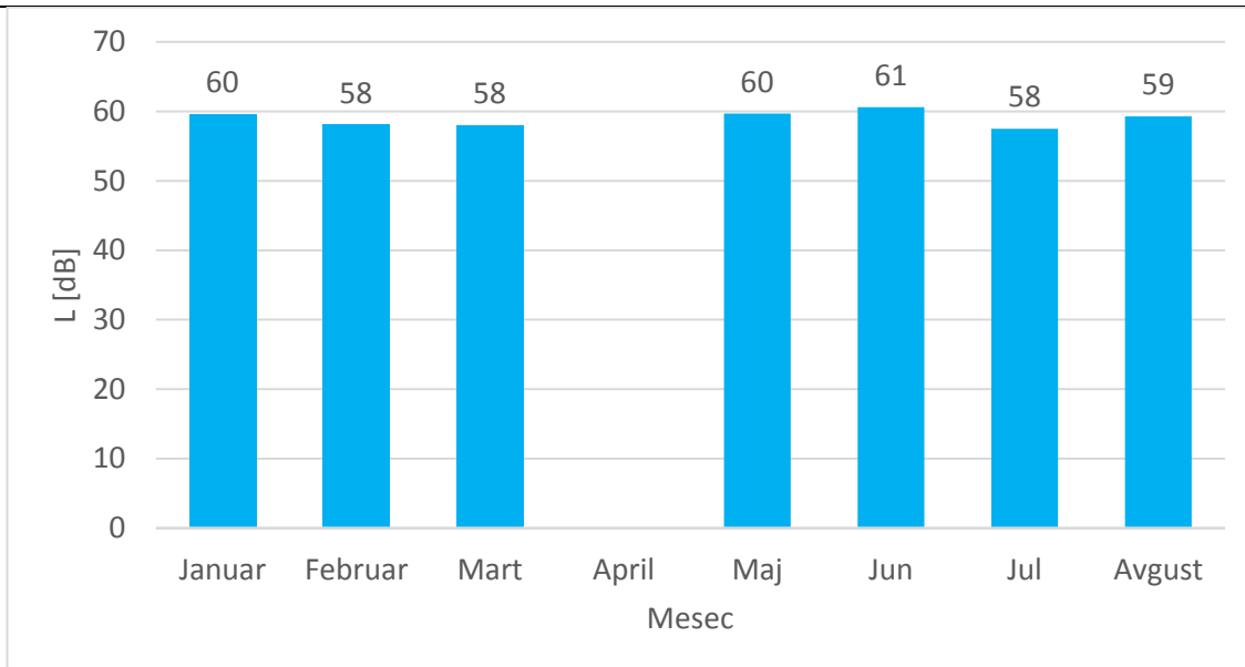
Slika MM7.3. Uporedni prikaz L day
