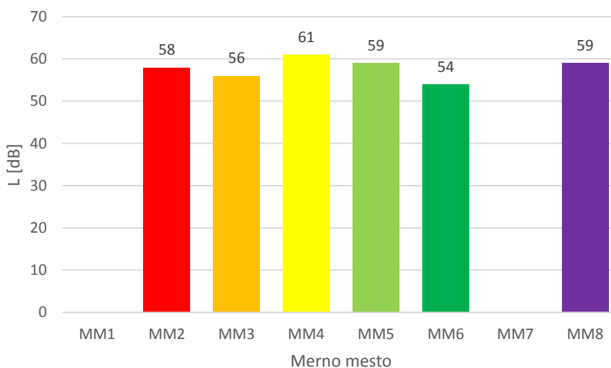
Slika 4.4. Ukupni nivo buke L_{den} – April 2020. godine
