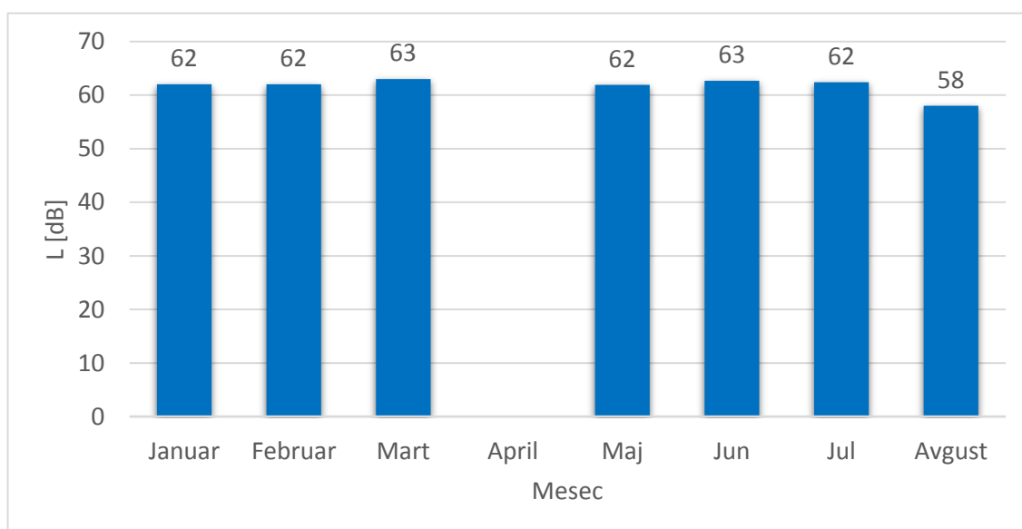
Slika MM1.6. Uporedni prikaz L_{den}
